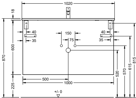
SHCB102
