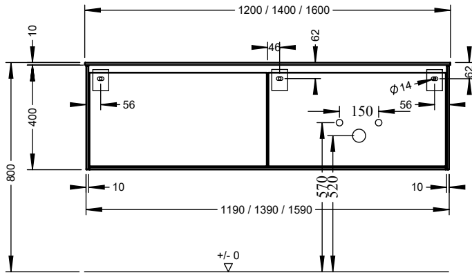
SGKN120R, SGKN140R, SGKN160R X = abhängig vom Waschtisch SGKP120R, SGKP140R, SGKP160R
